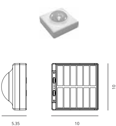
Solar Hybrid Module S (Couture S) Item Code : LP6533
